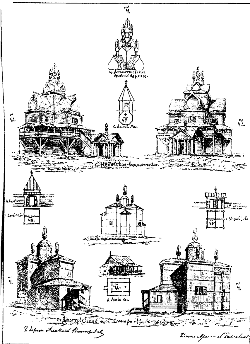
Ч. С. Нелазское и Борисоглѣбское 1674—1696 г. соврем. виды церкви (№ 38) Чл. Б. Дмитріевское или Старо-Никольское древн. многогл. верхъ и соврем. виды Церкви. (№ 37). Святыя ворота: 92. Чв. въ с. Дроздѣвъ (№ 89) и 92. Чв'. въ с. Муравѣвъ (№ 46). — Череповецкій у. 93 Чг. Часовня въ с. Ламской Пуст. (№ 48), гдѣ отдыхалъ некогда св. Кириллъ Бѣлозерскій. 94 Чл. Часовня въ д. Лемѣ (№ 83).
